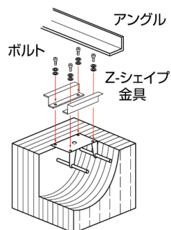
D・ブロック-S2 (ケーシングレスタイプ)
