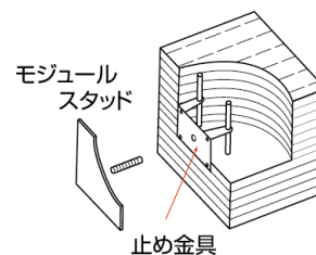
D・ブロック-T (内止めワンタッチタイプ側壁用)
