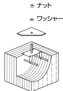
D・ブロック-S1 (外止めタイプ)
