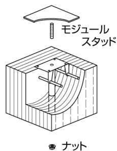
D・ブロック-B (内止めタイプ)
